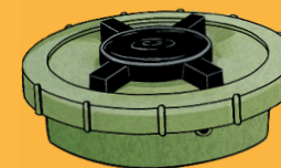
Противіхотна фугасна міна натискної дії
